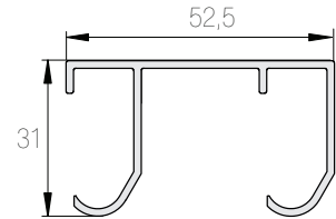
Sarja 40 K-40 (Al) Kantavuus 45 kg
