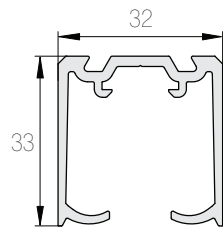
Sarja 75 K-75 Flow (Al) Kantavuus 100 kg
