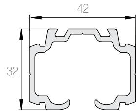
Sarja 75 K-75 P (Al) Kantavuus 100 kg
