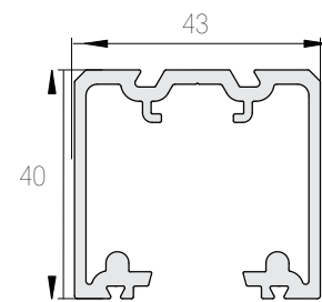
Sarja SAGA K-150/SAGA (Al) Kantavuus 150 kg
