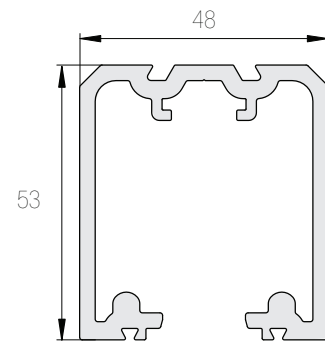
Sarja SAGA K-300/SAGA (Al) Kantavuus 300 kg
