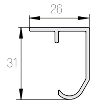
Sarja 30 K-30 (Al) Kantavuus 45 kg
