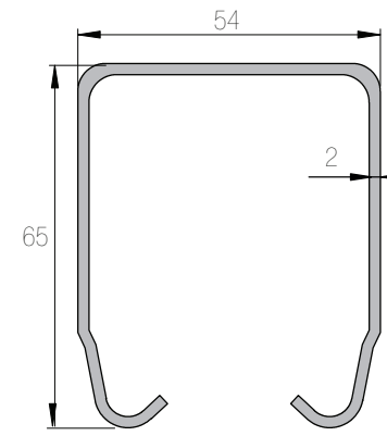
Sarja 300 K-300 Kantavuus 300 kg
