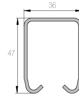
Sarja 150 K-150 Kantavuus 200 kg
