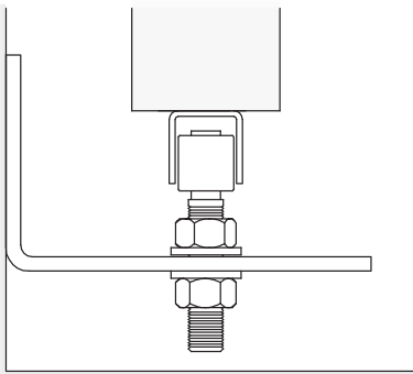
Alaohjainkisko on kiinnitetty oven pohjaan
