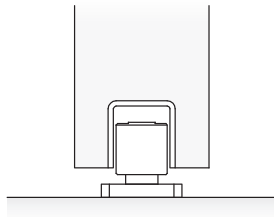
Alaohjainkisko on upotettu oven uraan
