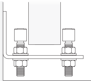
Ovi liikuu kahden alaohjainrullan välissä
